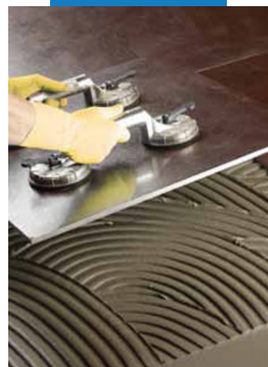
Укладка крупноформатного керамогранита на Kerabond T-R (Керабонд Т-Р) замешанный с Admix I
